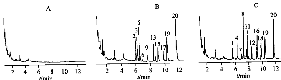
图 1 尿液提取物色谱图(非衍生化分析, HP-5 色谱柱)
